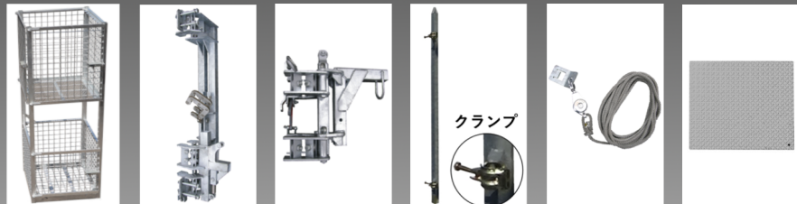
運搬カゴ ガイド材 ウインチ用ブラケット レール材 滑車・ロープ 敷板
